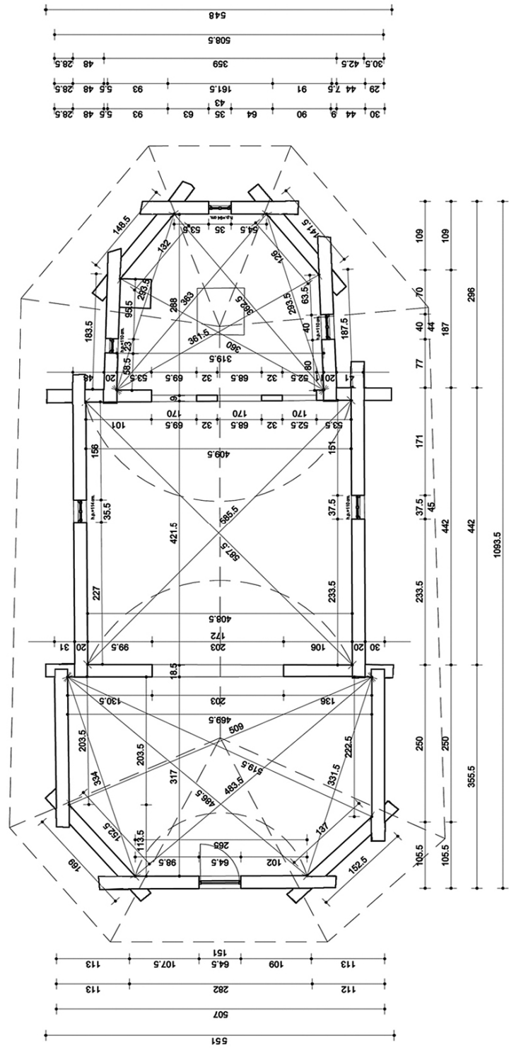
Biserica de lemn Sf. Nicolae din Pietrari-Angehești: plan și plan al tăpilor.
